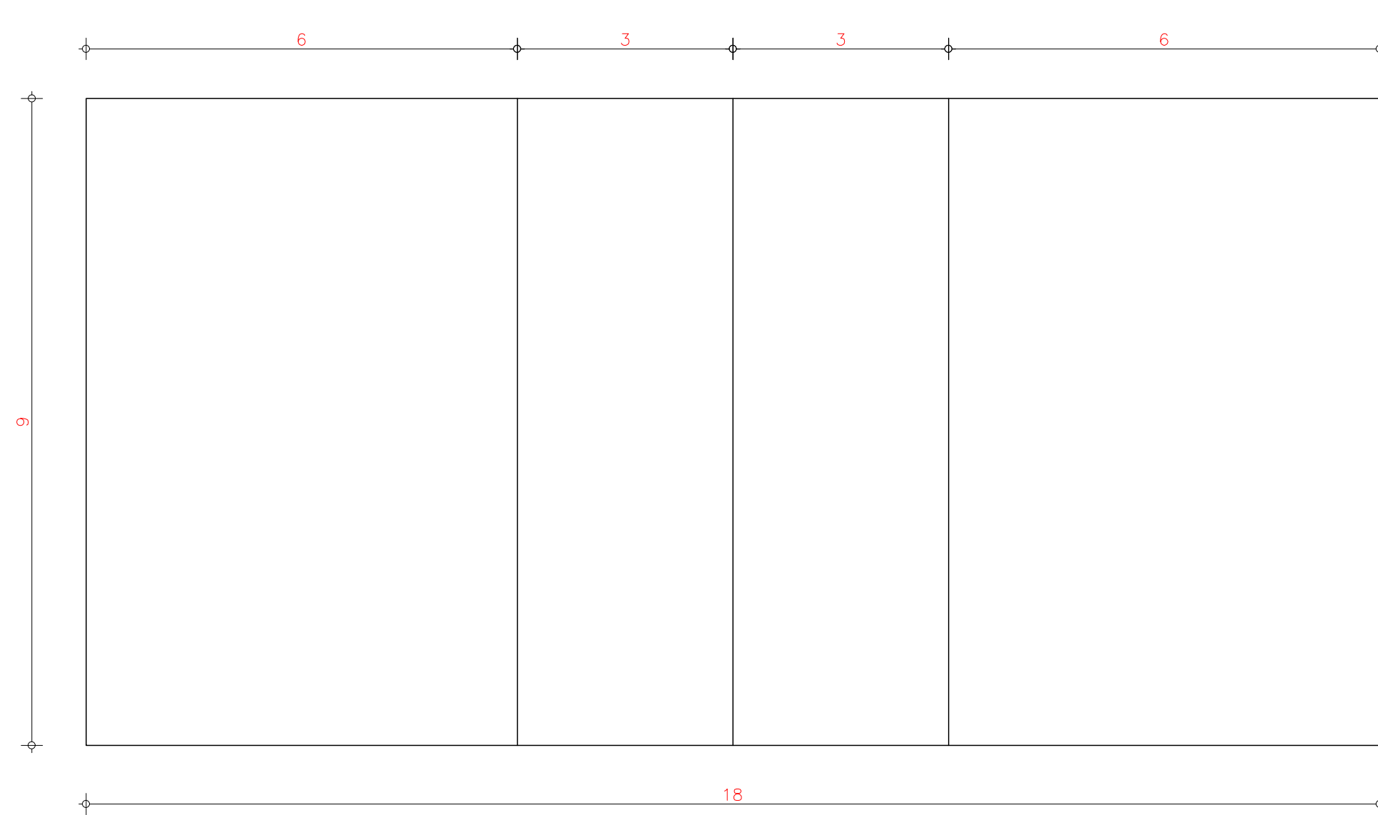
06 DEMARCAÇÃO - VOLEIBOL
