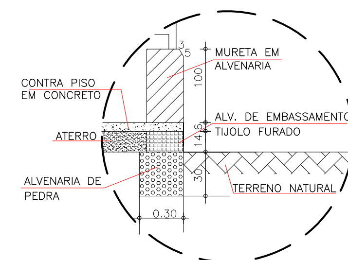
08 DETALHE - 01 E 02 esc: _____ 1/25
