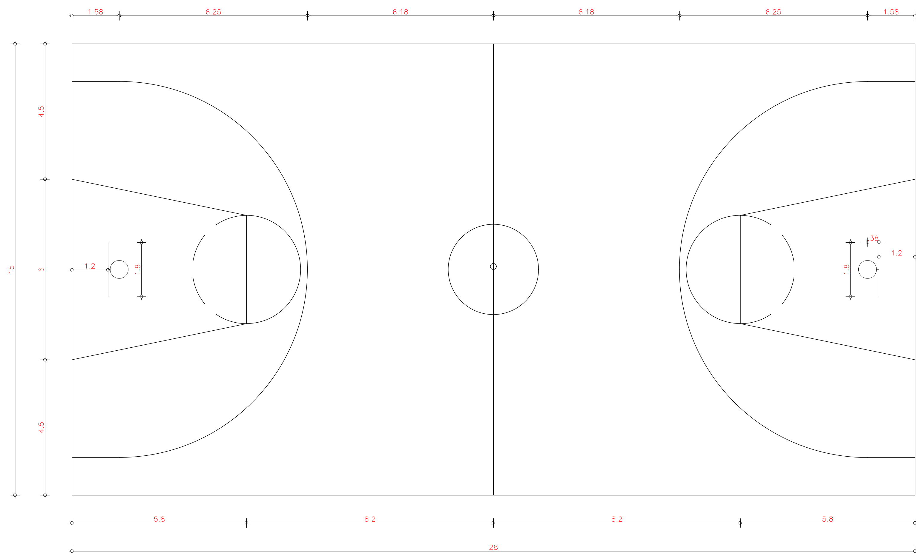
04 DEMARCAÇÃO - BASQUETBOL
