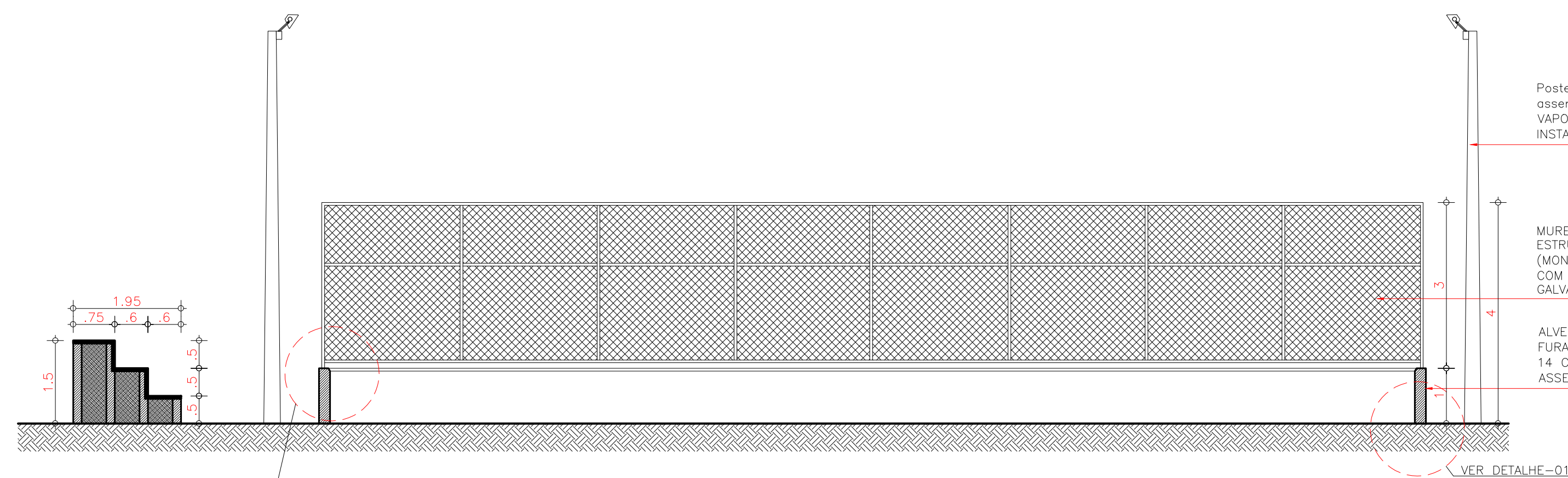
03 CORTE BB" esc: _____ 1/75
